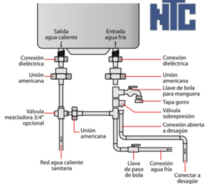
Esquema de instalación sugerida
